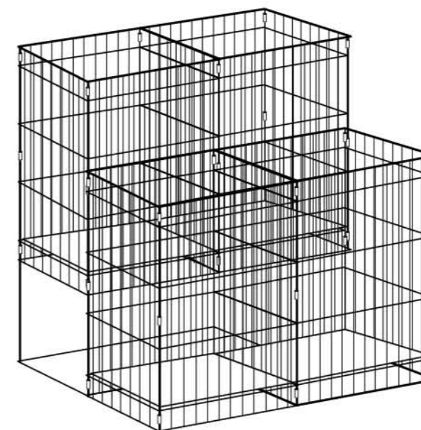
Typ: 9705-0002 Kapacita: 200 ks š/v/h: 59 / 91 / 47 / dodávaný v demonte/
